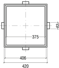
PLANTA TAPA CARA SUPERIOR
