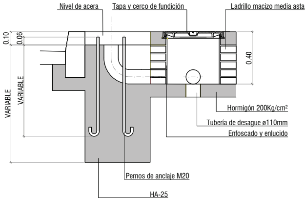
SECCION A-A
