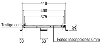
SECCION DE MARCO Y TAPA
